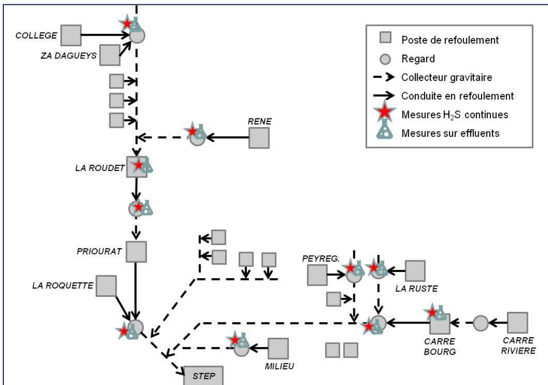
Figure 3 : Principe du réseau d’assainissement étudié
